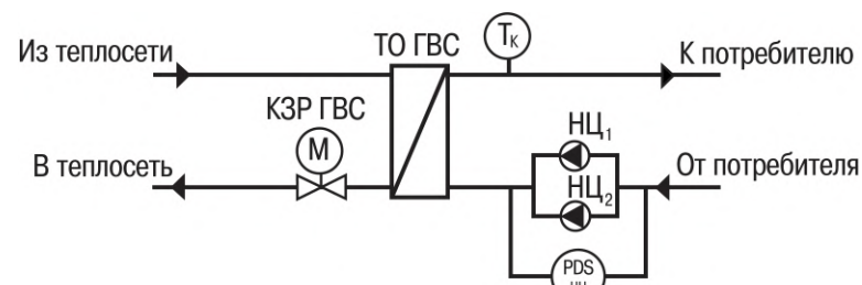
Рисунок 3.2 – Схема контура «ГВС»
