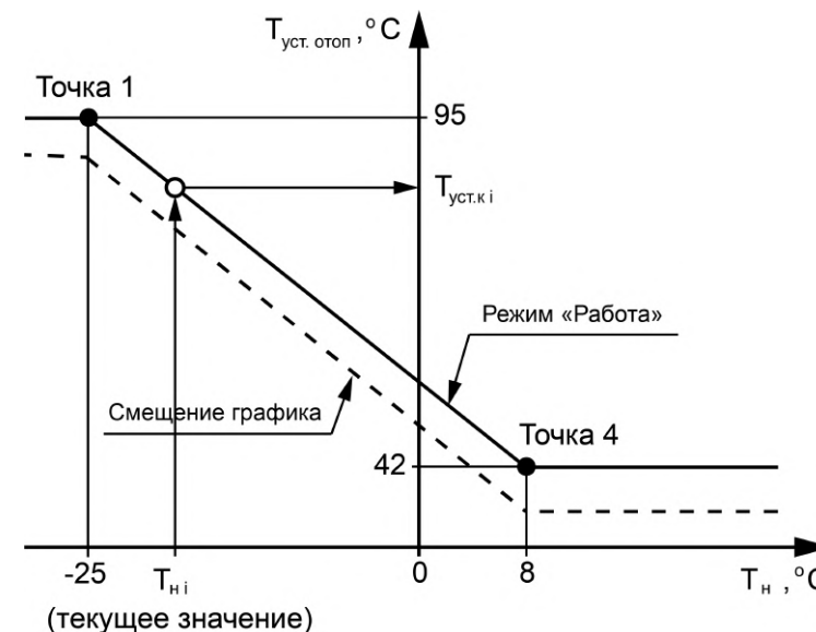
Рисунок 13.3 – Отопительный график
