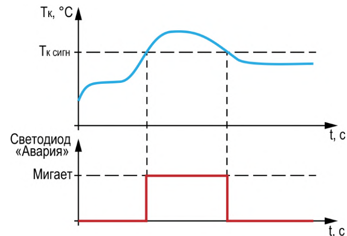
Рисунок 14.4 – Срабатывание светодиода «Авария»
