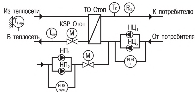
Рисунок 3.1 – Схема контура «Отопление»
