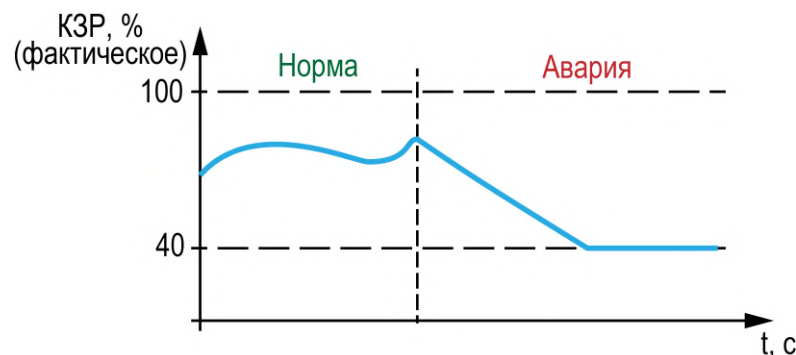
Рисунок 14.3 – Работа КЗР – норма/авария
