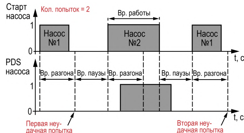
Рисунок 14.8 – Перезапуск насоса
