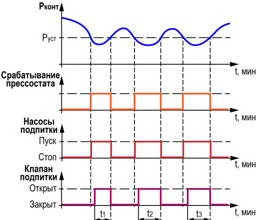
Рисунок 13.12 – Работа насосов и клапана подпитки
